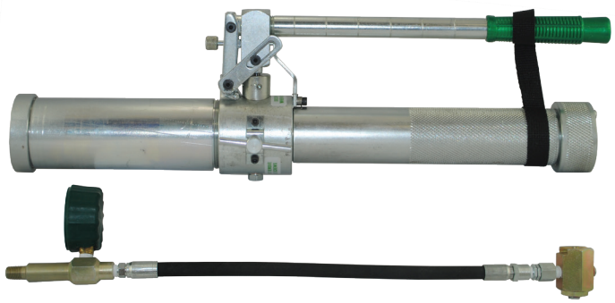
Pistola manual hidráulica de alta presión GRM (manguera articulada de 16")
